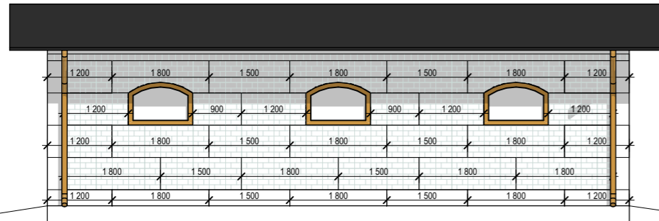
FASAD LÅNGSIDA 33 BLOCK X 1 SIDA
