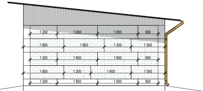
FASAD KORTSIDA 20 BLOCK X 2 SIDOR
